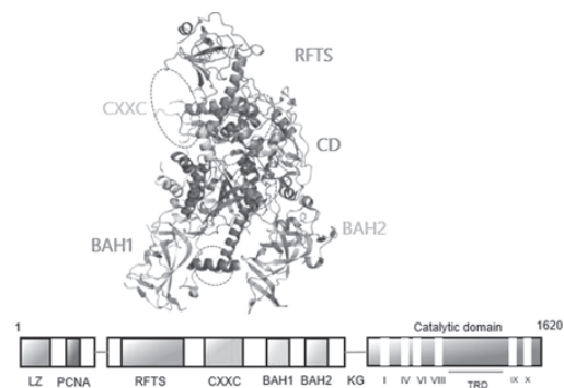
図4 マウス Dnmt1
